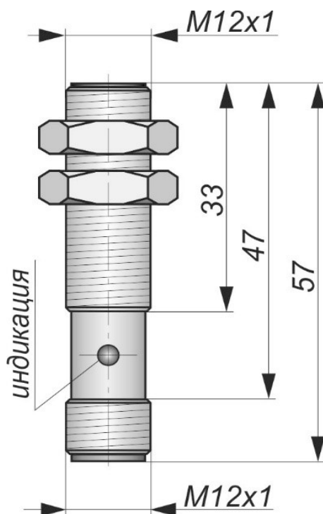
Габаритный чертеж
