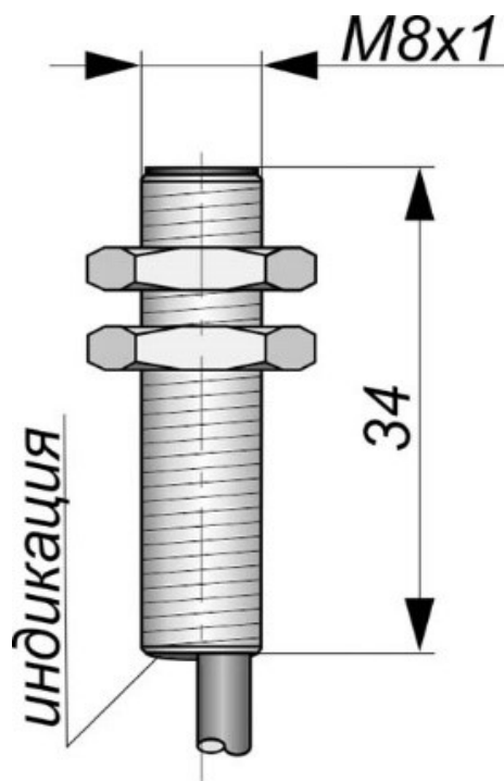
Габаритный чертеж
