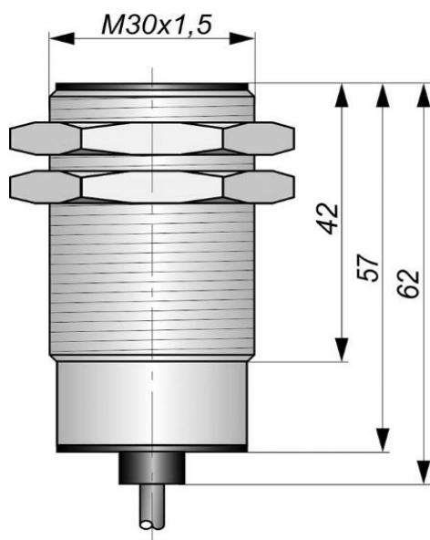
Габаритный чертеж
