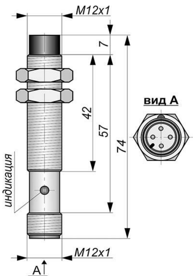
Габаритный чертеж
