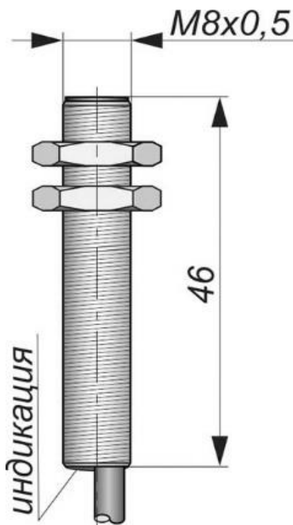
Габаритный чертеж
