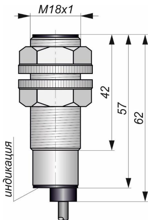
Габаритный чертеж
