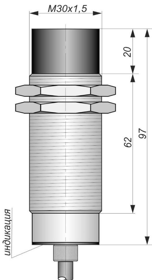
Габаритный чертеж
