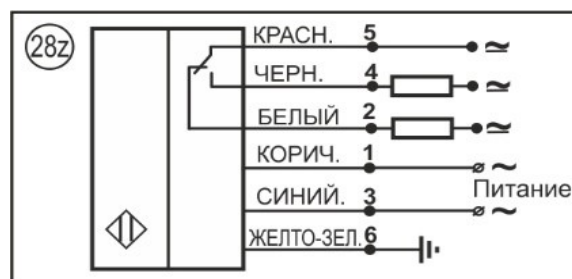
Схема соединения
