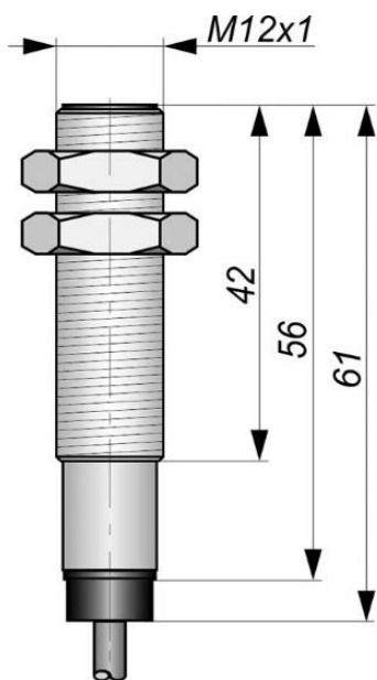
Габаритный чертеж
