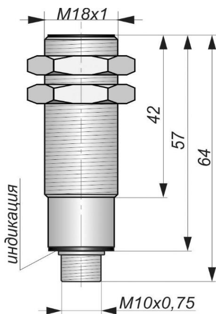
Габаритный чертеж
