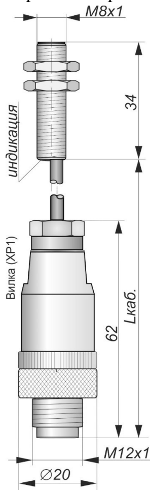
Габаритный чертеж
