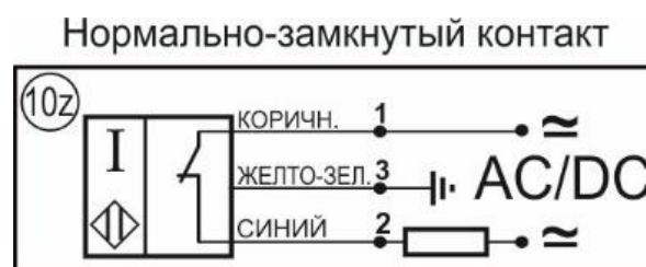
Схема соединения
