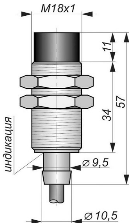
Габаритный чертеж
