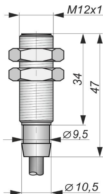
Габаритный чертеж
