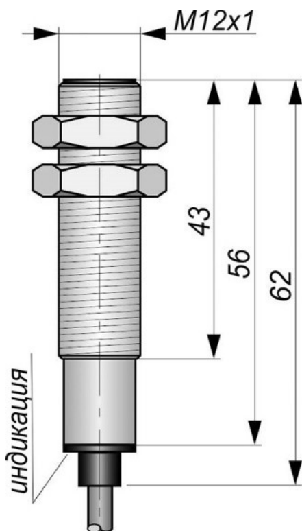
Габаритный чертеж
