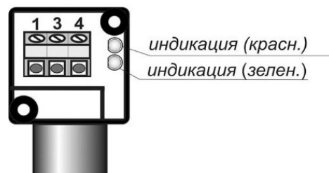
Цоколевка клеммной колодки
