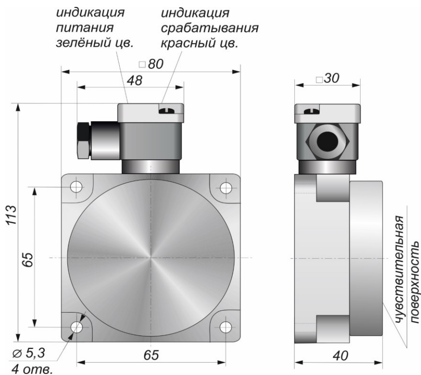
Габаритный чертеж
