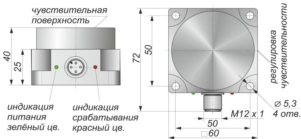
Переключающий контакт
