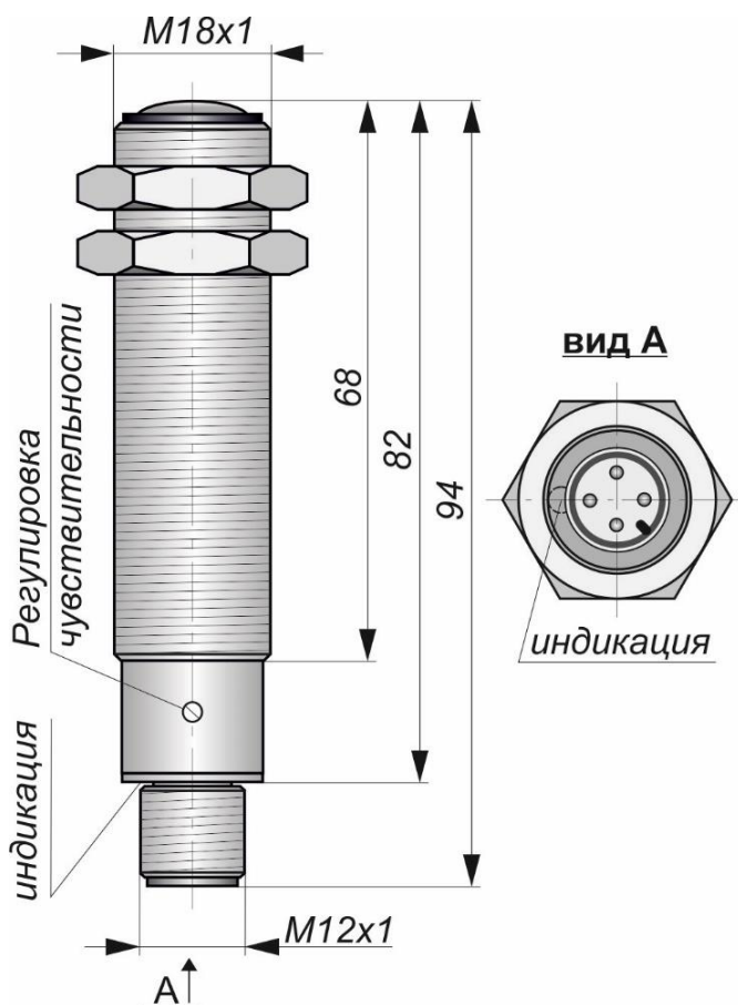
Габаритный чертеж
