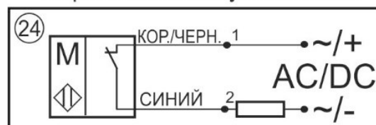
Схема соединения
