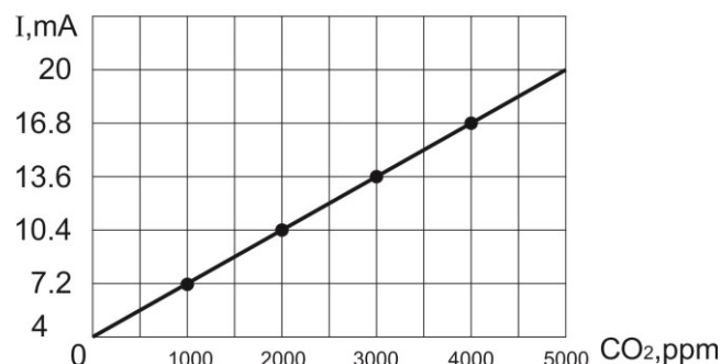
Выходная характеристика анализатора
