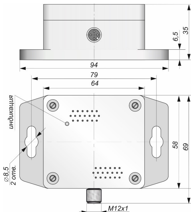
Габаритный чертеж
