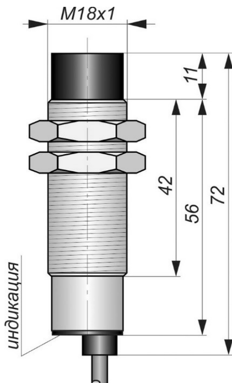
Габаритный чертеж
