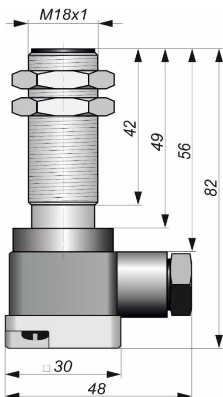
Габаритный чертеж
