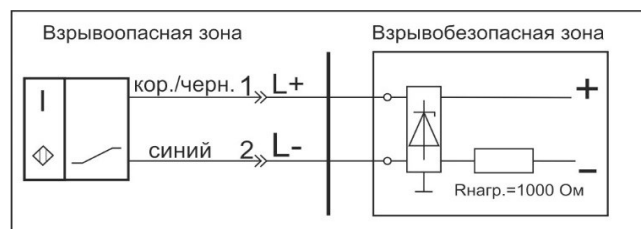
Цоколевка клеммной колодки
