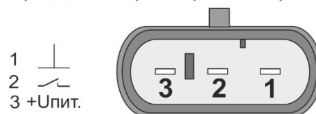
Схема соединения
