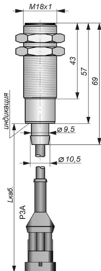
Габаритный чертеж
