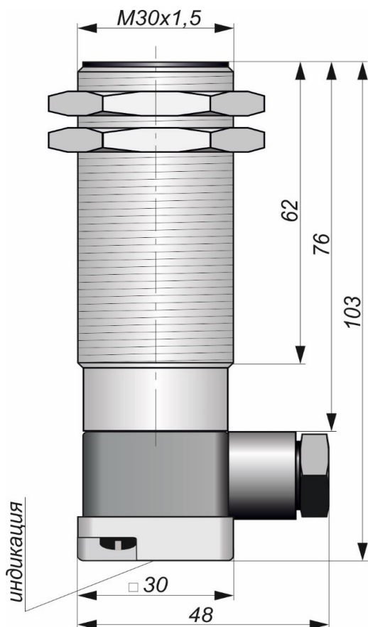
Габаритный чертеж
