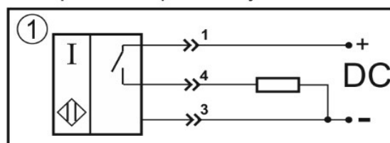
Нормально-разомкнутый контакт
