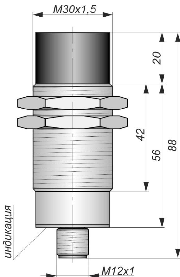
Габаритный чертеж
