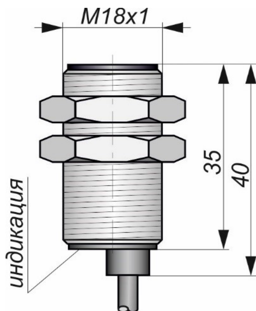
Габаритный чертеж
