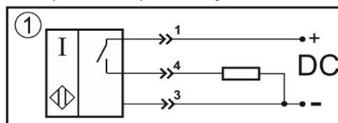
Цоколевка разъема
