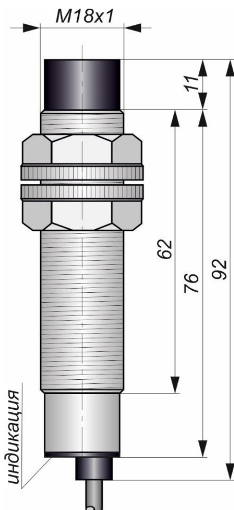
Габаритный чертеж
