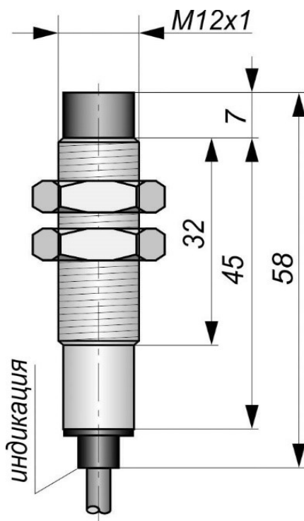
Габаритный чертеж
