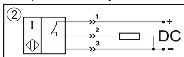
Нормально-замкнутый контакт
