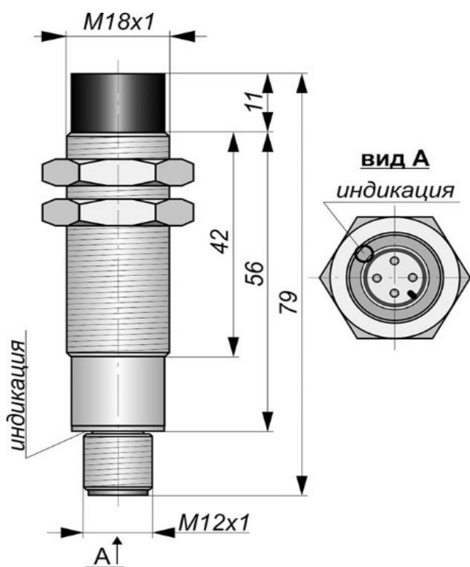
Габаритный чертеж
