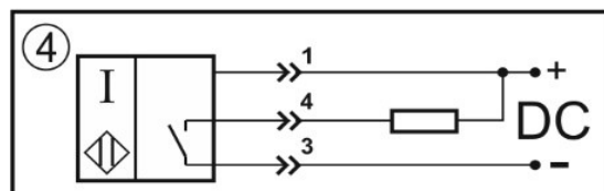
Нормально-разомкнутый контакт
