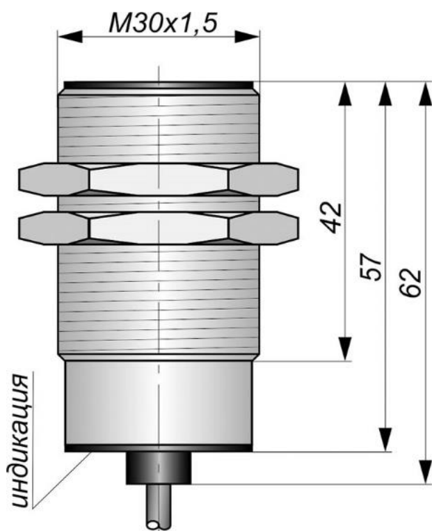
Габаритный чертеж
