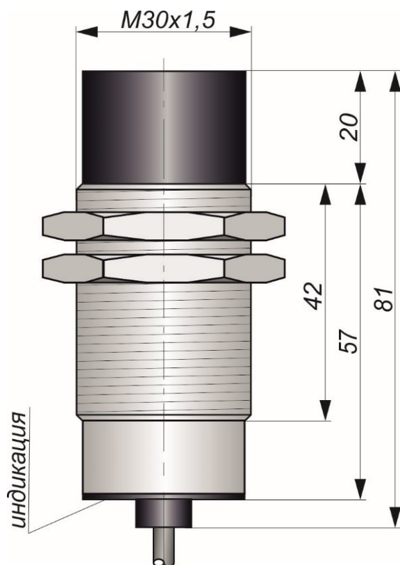
Габаритный чертеж
