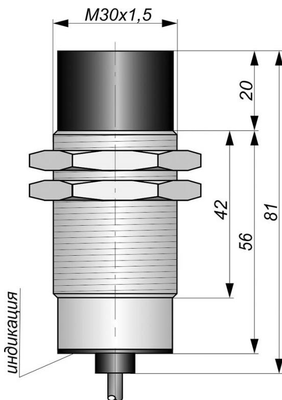
Габаритный чертеж
