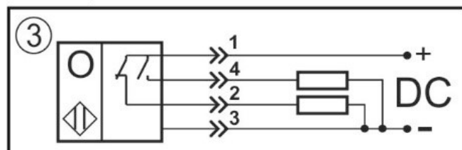
Переключающий контакт
