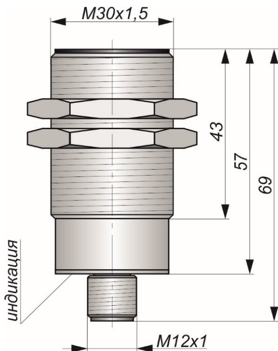
Габаритный чертеж
