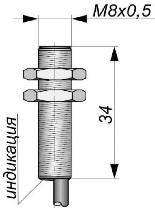
Габаритный чертеж
