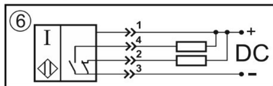
Переключающий контакт
