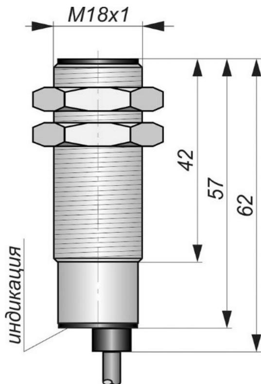
Габаритный чертеж
