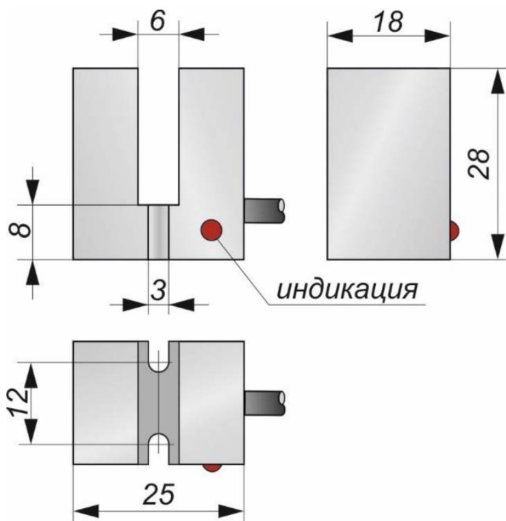
Габаритный чертеж
