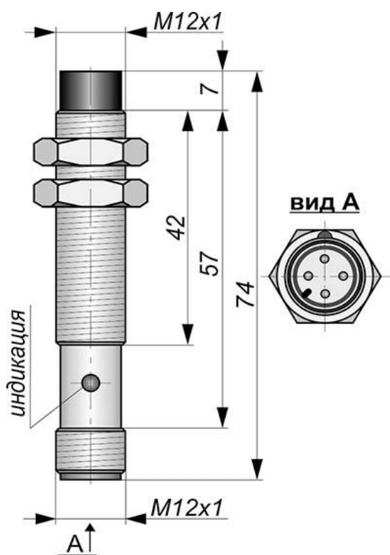
Габаритный чертеж
