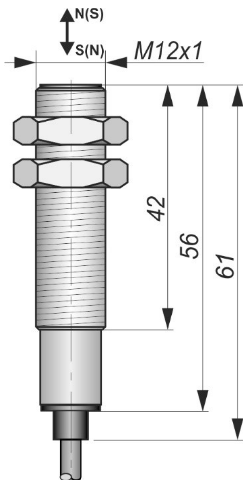
Габаритный чертеж
