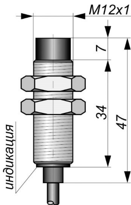
Габаритный чертеж
