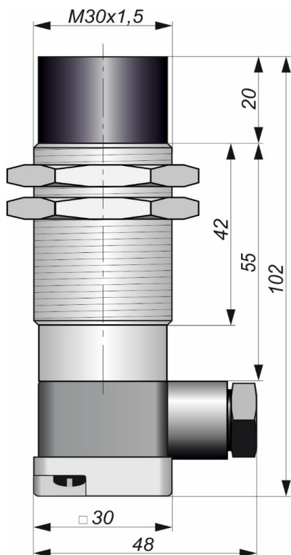
Габаритный чертеж
