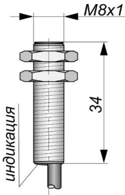
Габаритный чертеж
