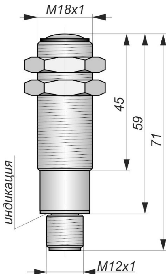
Габаритный чертеж
