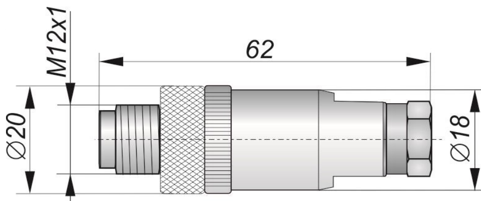
Габаритный чертеж
