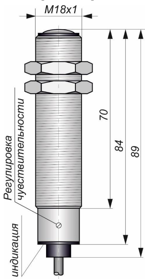
Габаритный чертеж
