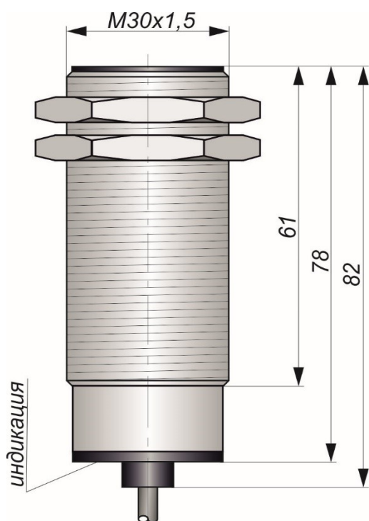
Габаритный чертеж
