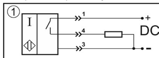
Цоколевка разъема
