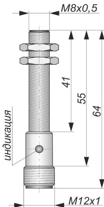
Габаритный чертеж
