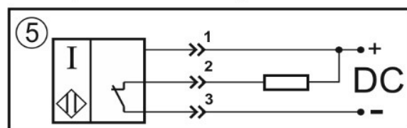
Нормально-замкнутый контакт
